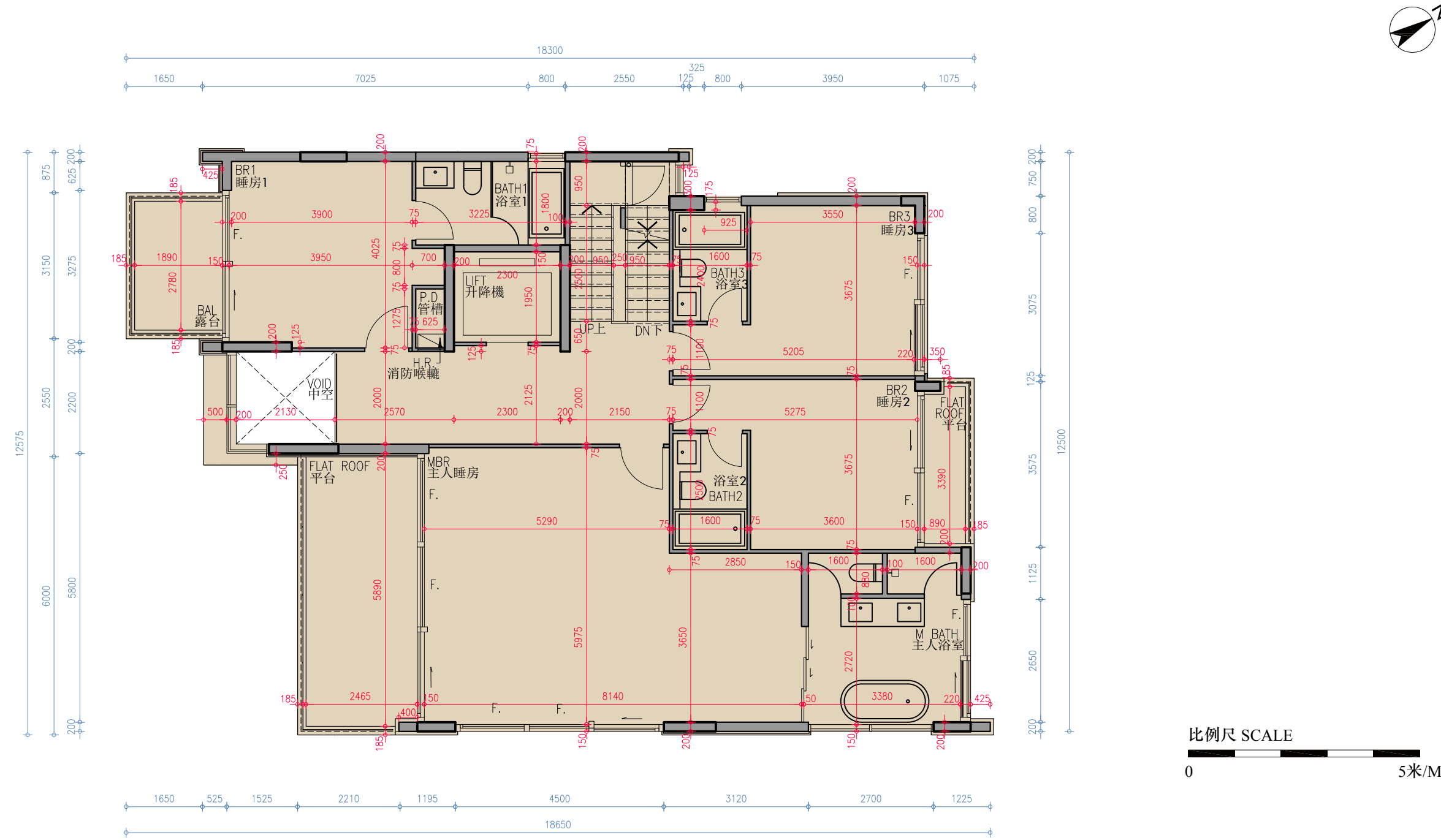
1 號洋房 1 樓平面圖 HOUSE 1 FIRST FLOOR PLAN
