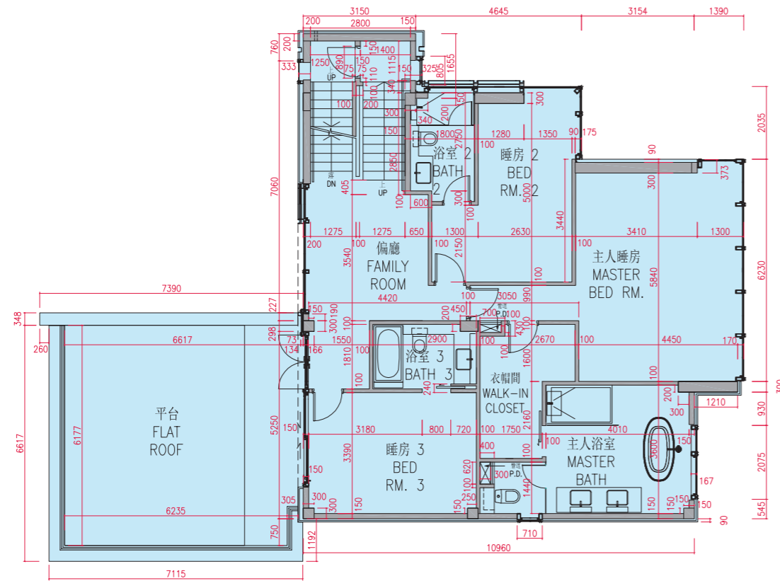
一樓平面圖 1/F FLOOR PLAN
