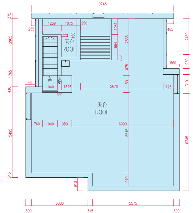
天台平面圖 ROOF FLOOR PLAN
