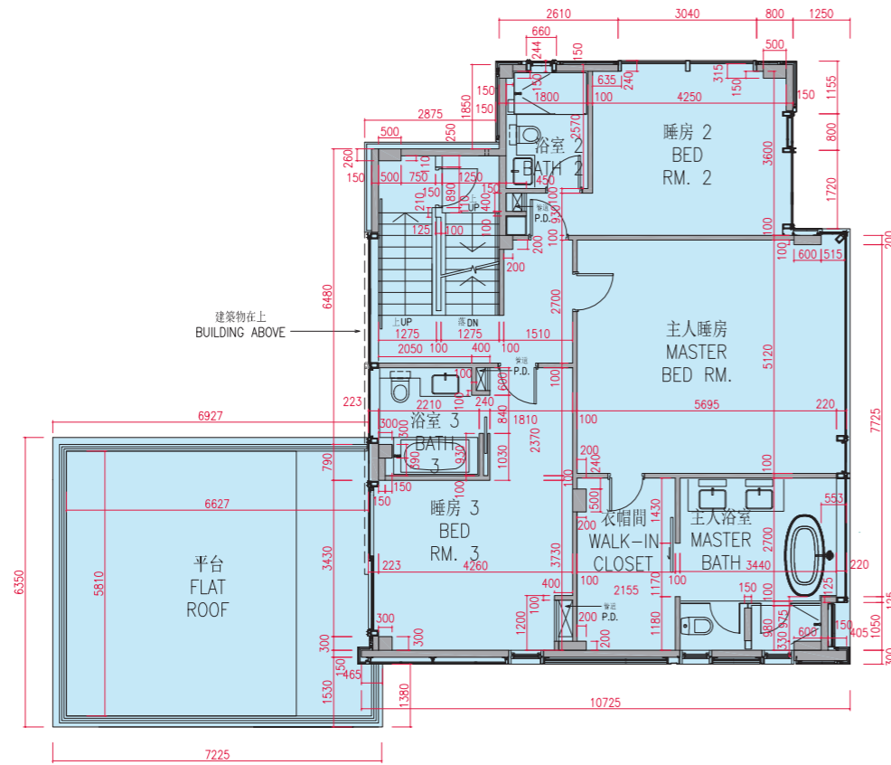
一樓平面圖 1/F FLOOR PLAN
