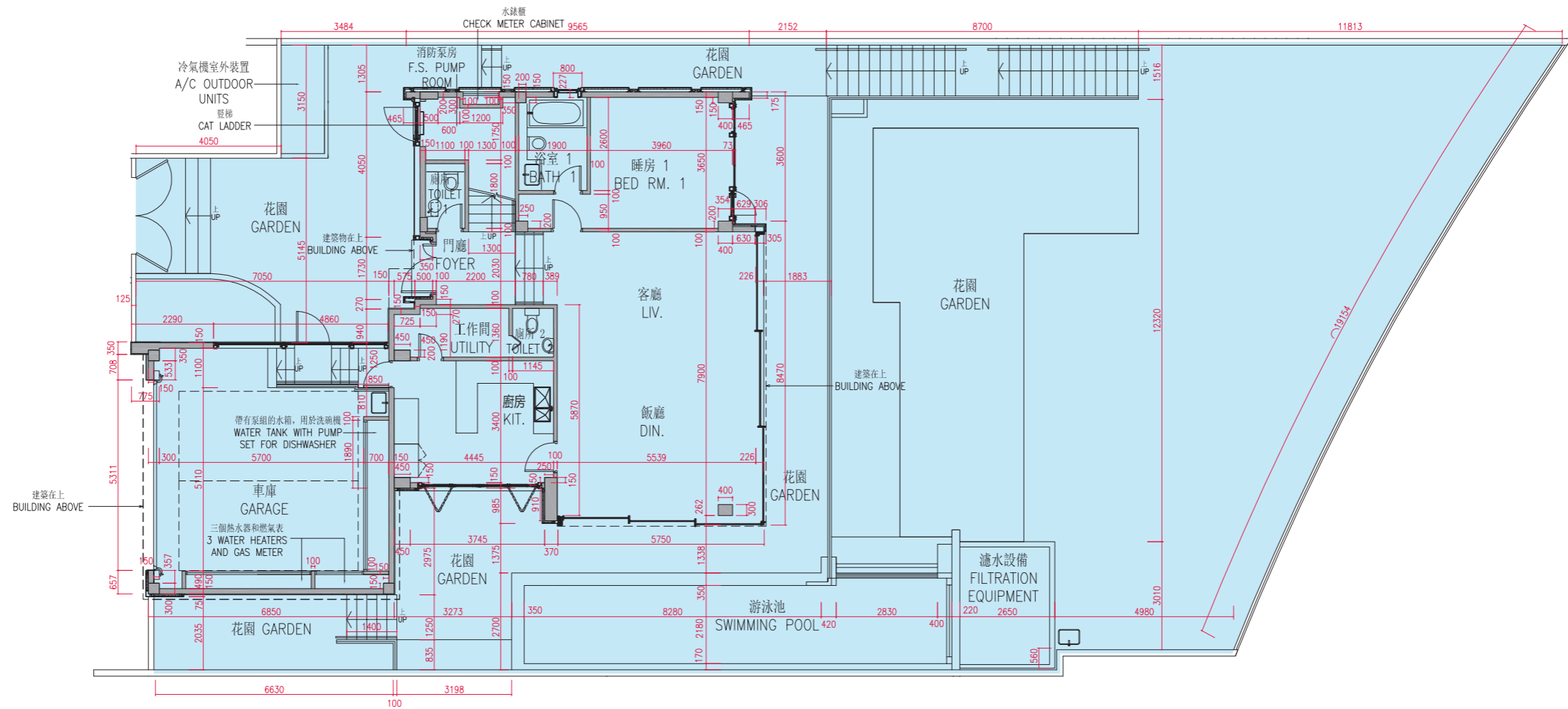
地下平面圖 G/F FLOOR PLAN
