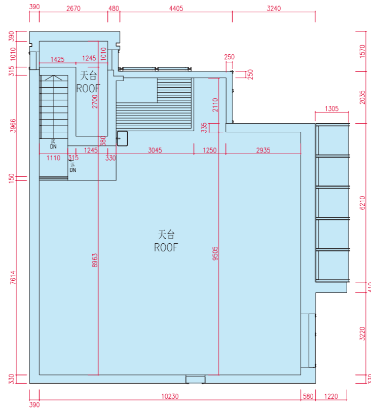
天台平面圖 ROOF FLOOR PLAN
