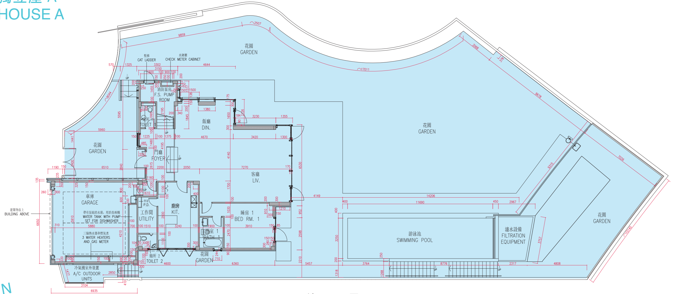
地下平面圖 G/F FLOOR PLAN
